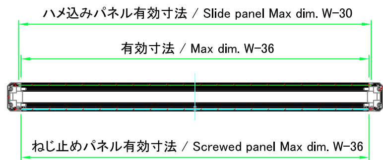
A-A (1:5)
